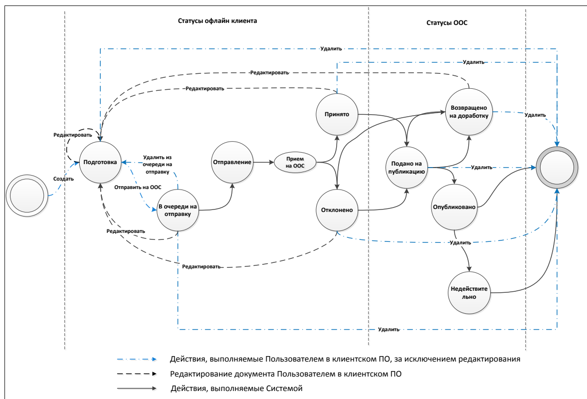
Рис. 1 – Схема жизненного цикла сведений версии плана-графика
